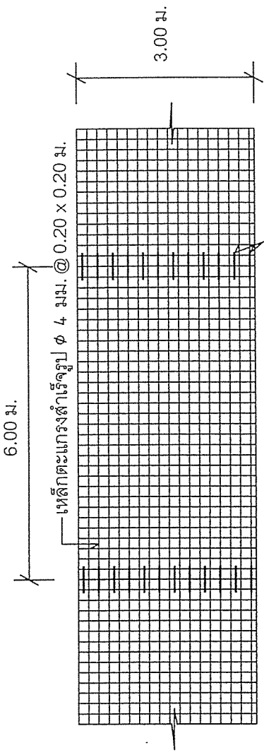
แปลนแสดงการเสริมเหล็กถนนคอนกรีต
